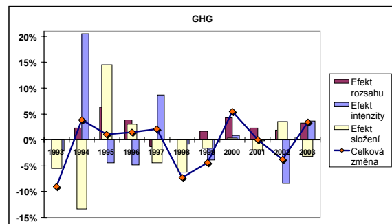
Obrázek 5 : Efekty rozsahu složení a intenzity pro GHG
