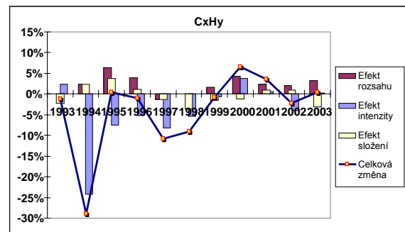
Obrázek 4 : Efekty rozsahu složení a intenzity pro CH
