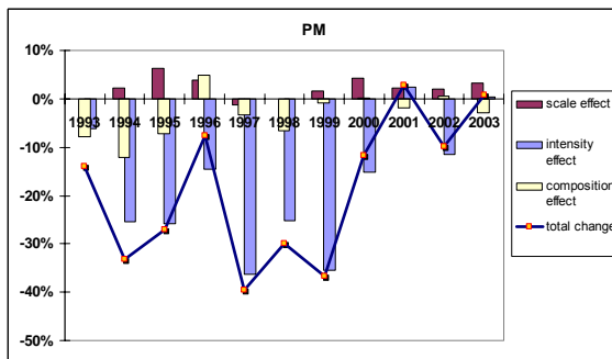
Obrázek 1 : Efekty rozsahu složení a intenzity tuhých znečišťujících látek
