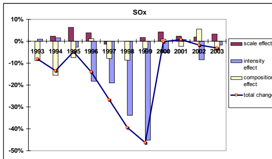
Obrázek 1 : Efekty rozsahu složení a intenzity pro SOx.
