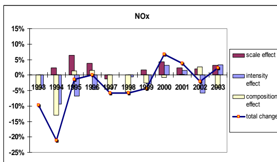
Obrázek 2 : Efekty rozsahu složení a intenzity pro NOx
