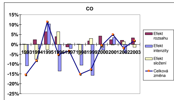
Obrázek 3 : Efekty rozsahu složení a intenzity pro CO
